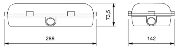
Montaje estanco
